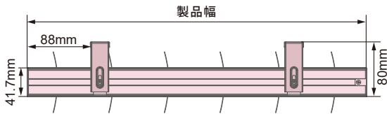
▲ 壁面付け
