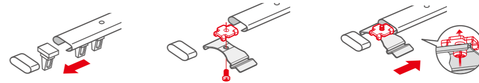
カーテンレールからランナーを外す ▶ ネジで仮止め ▶ 隙間を利用しレールにスライドさせる
