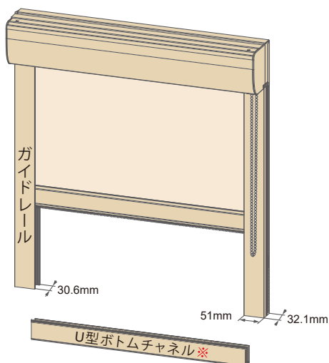
【チェーンタイプ】
