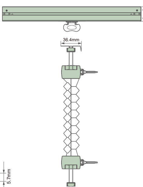
セルタイプ45D断面図
