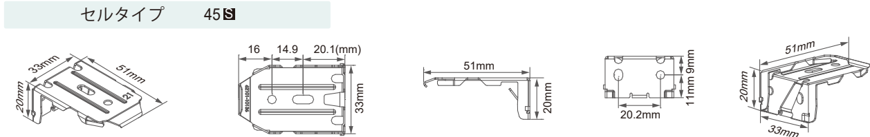
セルタイプ45S拡大イメージ図 ※生地とセルタイプは次のページをご確認ください。
