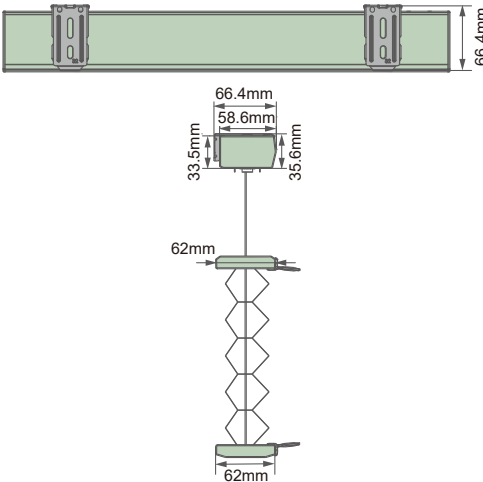
セルタイプ62S 断面図
