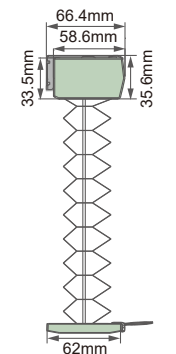
セルタイプ 62S 断面図
