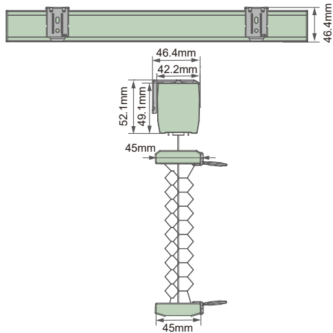
セルタイプ45D 断面図
