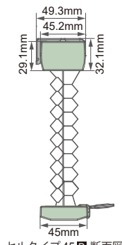
セルタイプ 45D 断面図
