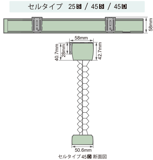
セルタイプ45D 断面図
