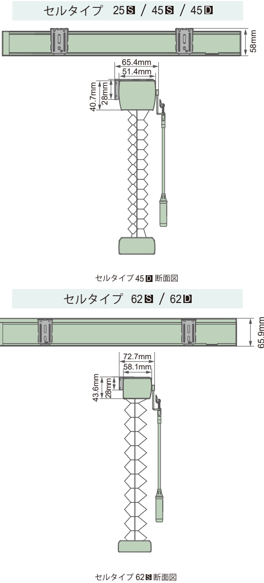
セルタイプ 62S 断面図
