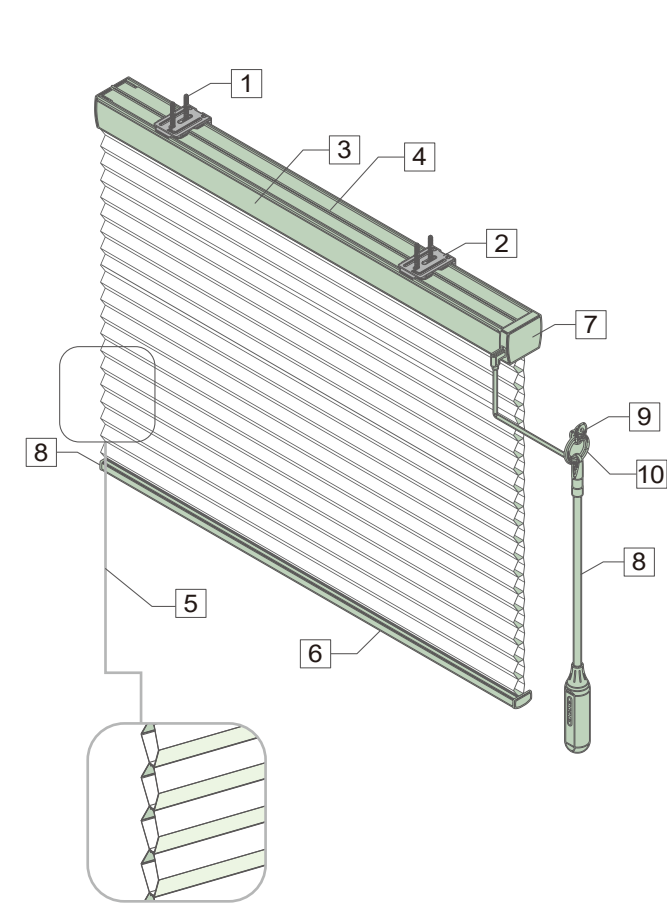
セルタイプ25S拡大イメージ図
