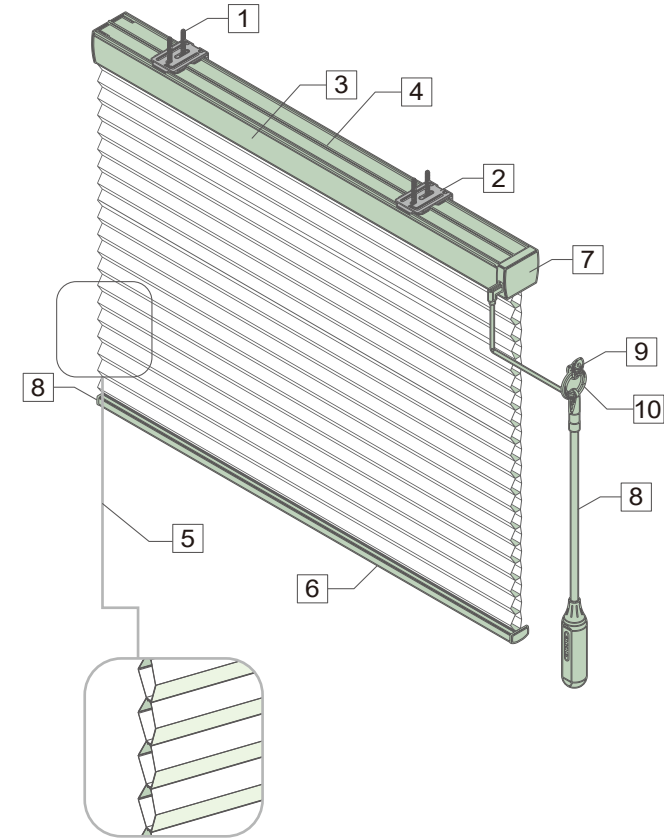
セルタイプ25S拡大イメージ図 ※ 生地とセルタイプは次のページをご確認ください。
