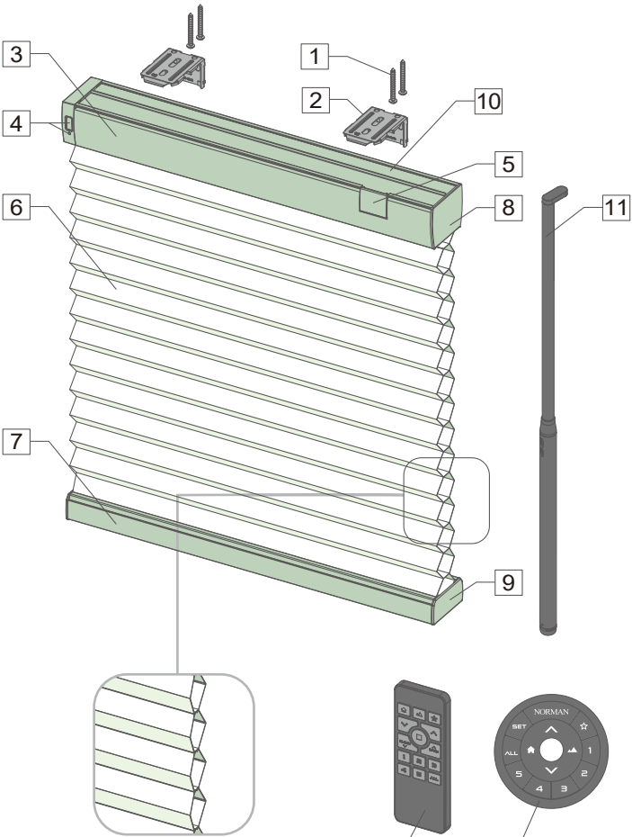
セルタイプ45S拡大イメージ図
