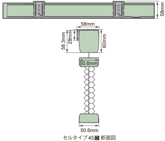
セルタイプ45D 断面図
