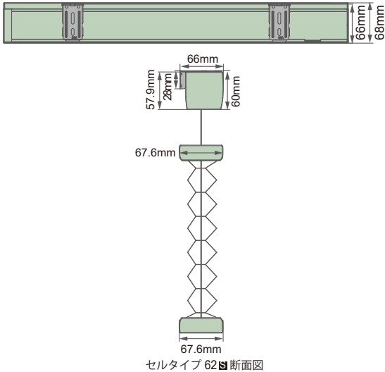
セルタイプ62S 断面図
