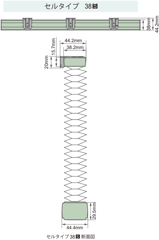
セルタイプ 38S 断面図
