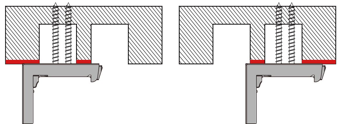
取り付けの側面図 (おすすめの取り付け方法)
